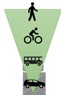
Figur 4 Ønsket transporthierarki
